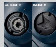
TWIN CANT PLUS システム アウトサイドにはカント調整機構、インサイド側には簡易型調整機構を採用して軽量化を実現。 R-EVO PLUS 100 以上モデルに採用。
